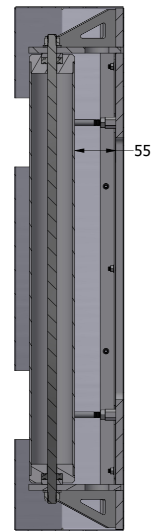
SECTION D-D SCALE 0,20 : 1
